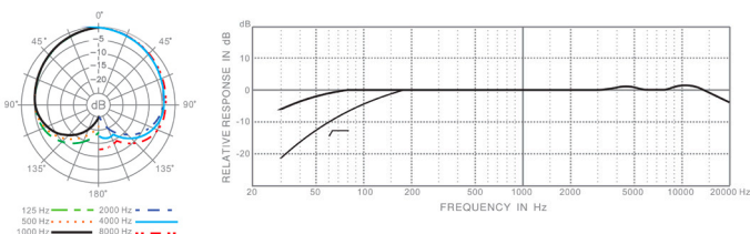
L211 頻率響應圖（心型）
