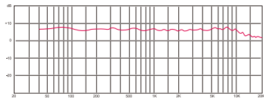
CM9HL频率响应图（超心型）
