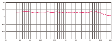
CM9HL頻率響應圖（超心型）
