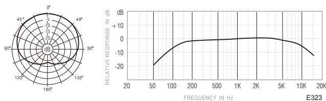
E323 频率响应图（心型）
