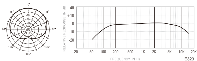
E323 頻率響應圖（心型）
