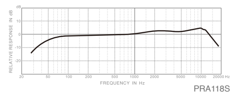
PRA118 頻率響應圖（槍型）
