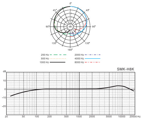
SMKH8K 频率响应图
