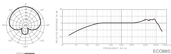
EC088S 頻率響應圖（超心型）
